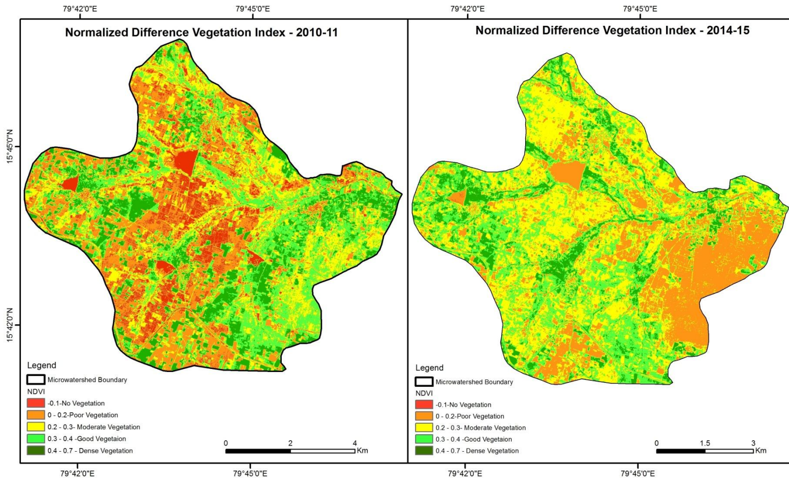
NDVI-2010-11
